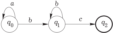
Рис. 8. Граф состояний автомата A_{x1}
