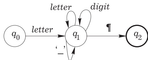
Рис. 7. Граф состояний автомата A_4
