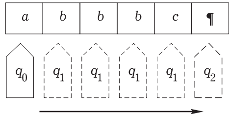
Рис. 3. Разбор автоматом A_1 строки « abbbc »
