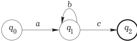
Рис. 2. Граф состояний автомата A_1
