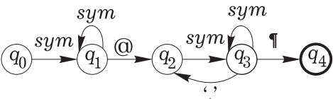
Рис. 9. Граф состояний автомата A_{x2}
