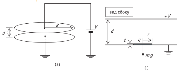
Рисунок 1.1 Схематический чертеж параллельных пластин конденсатора, подключенных к источнику постоянного напряжения, (a) и вид сбоку параллельных пластин с маленьким диском, помещённым внутри конденсатора (b). (Смотри подробное описание в тексте).
